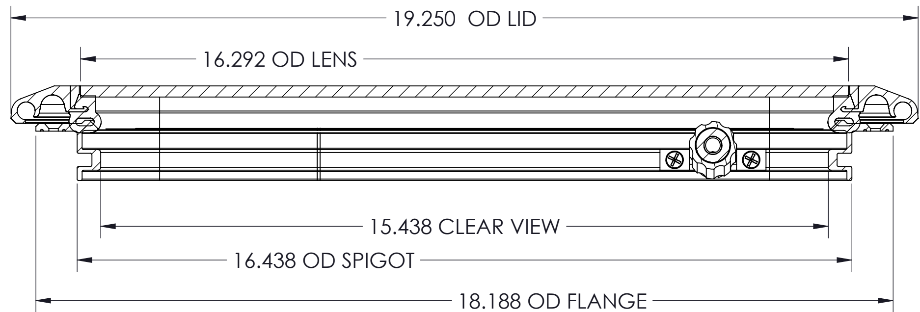
SECTION A-A
